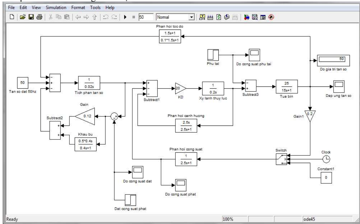
Hình 2.13. Sơ đồ mô phỏng bộ điều tốc khi cho đồng thời phụ tải, phản hồi công suất, và giá trị đặt phụ tải cùng tác động
