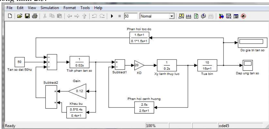
Hình 2.5. t tốc ở chế độ không tải
